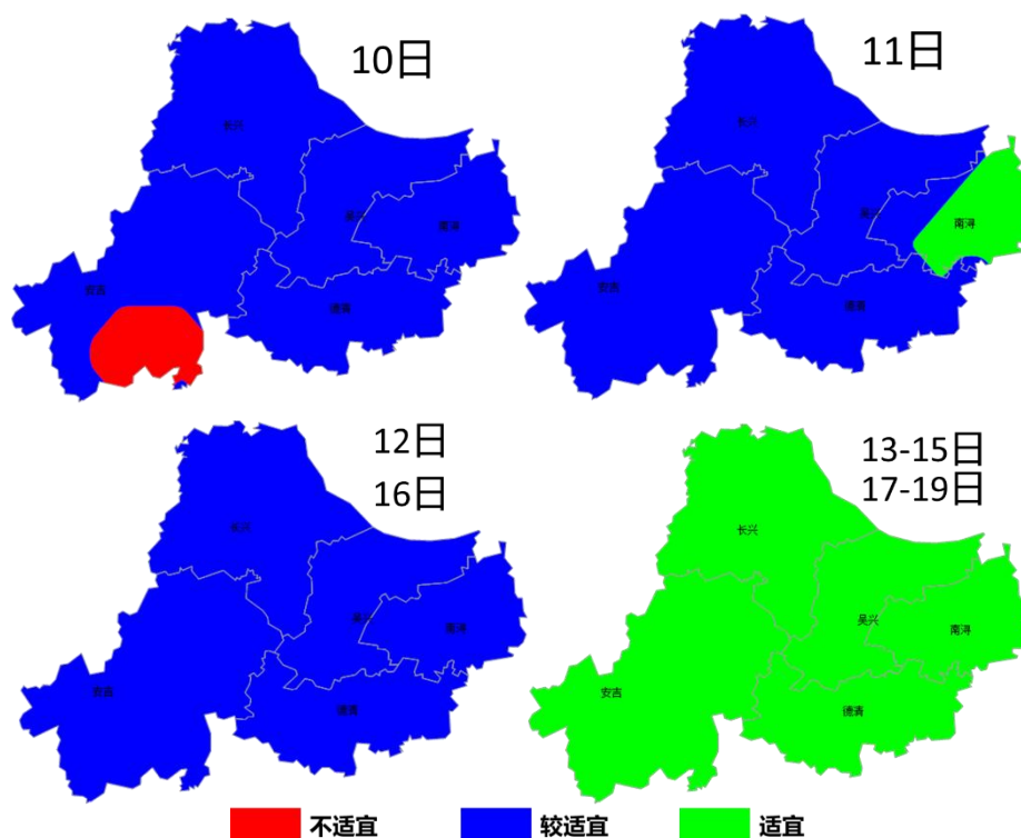
图1 11月10-19日湖州市单季晚稻收割适宜度
